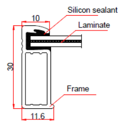
短边截面
