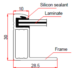
长边截面
