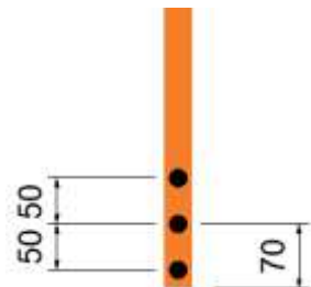
Configuration avec 3 vis de fixation rail / panneau sandwich par fixation universelle ou fixation extérieure
