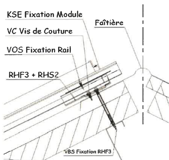
Positionnement des rehausses de faîtage : une seule par colonne de rails
