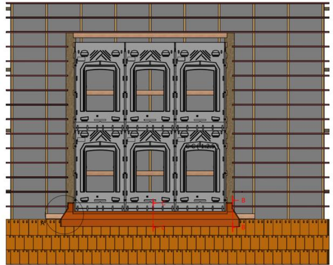
Pose de la bande au niveau du couloir
