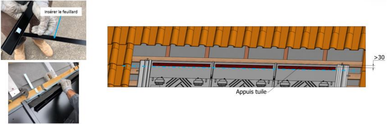
Figure 26 – Pose des appuis de tuiles (kit TS-2)
