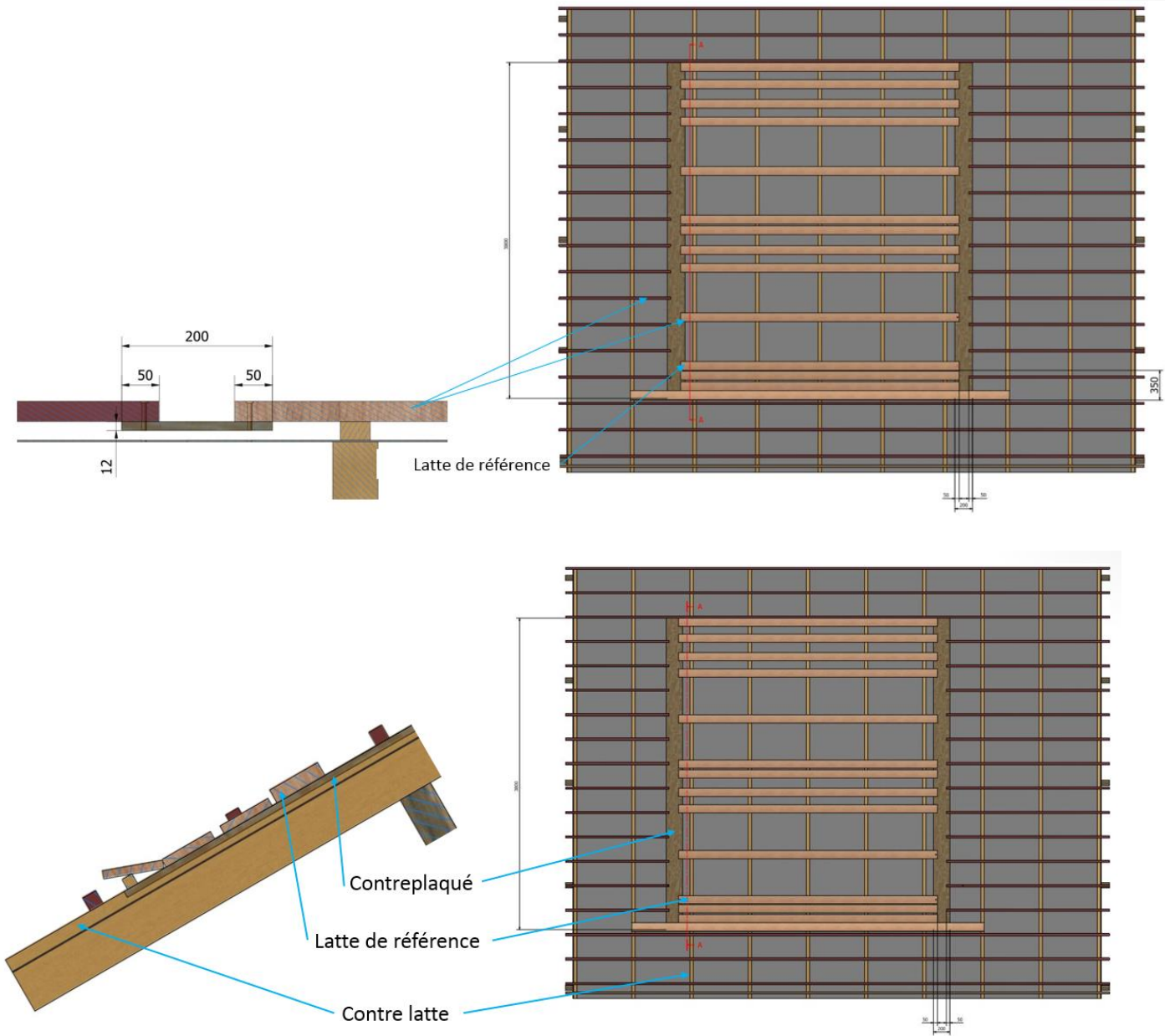
Figure 35 – Pose de la fonçure (kit TN-1)
