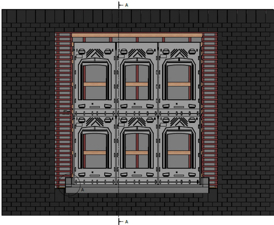
Figure 30 – Mise en œuvre du bas de champ (kit A-2)
