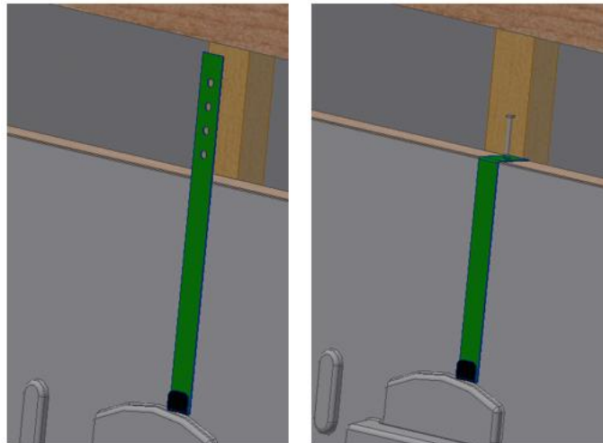
Figure 24 – Pose des abergements supérieurs (kit TS-2)
