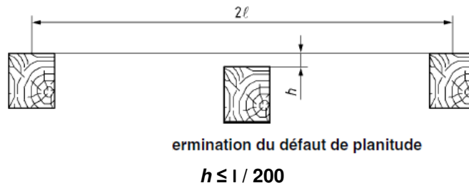
Figure 15 – Contrôle de la planitude
