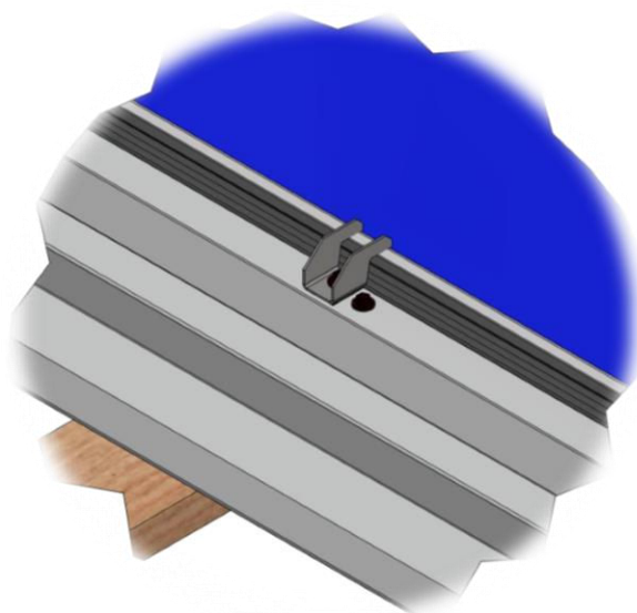
D : Placer le module et fixer les nouveaux ensembles (étrier + joint EPDM + vis CAPINOX).
