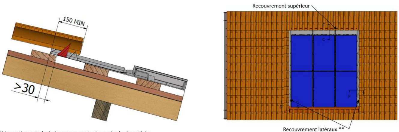
Figure 28 – Mise en place des éléments de couverture (kit TS-2)
