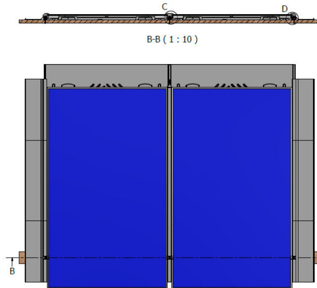
Figure 21 – Exemples de chaînes de cotes de l'écrasement du joint EPDM sous les étriers
