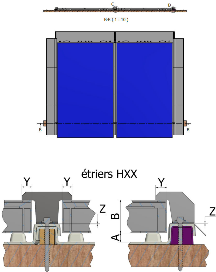
Figure 21 – Exemples de chaines de cotes de l'écrasement du joint EPDM sous les étriers
