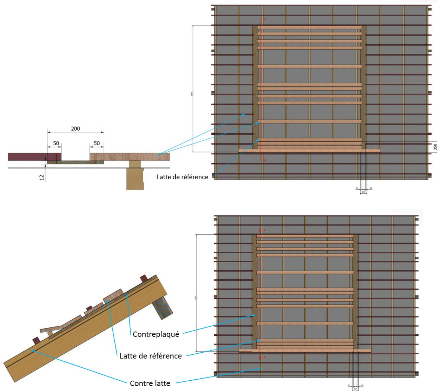
Figure 35 – Pose de la fonçure (kit TN-1)
