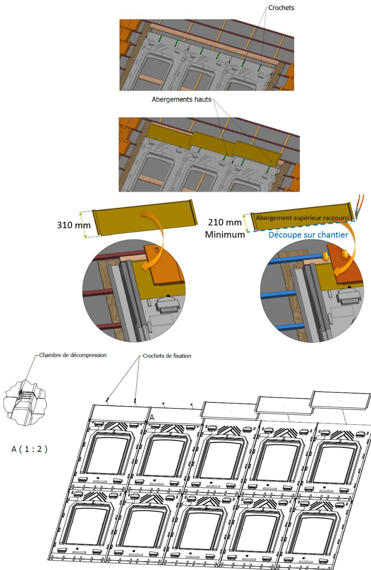
Figure 37 – Pose des abergements supérieurs (kit TN-1)
