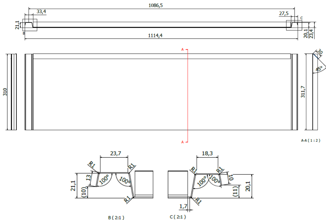
Figure 7 – Abergements supérieurs kits TS-2 et TN-1
