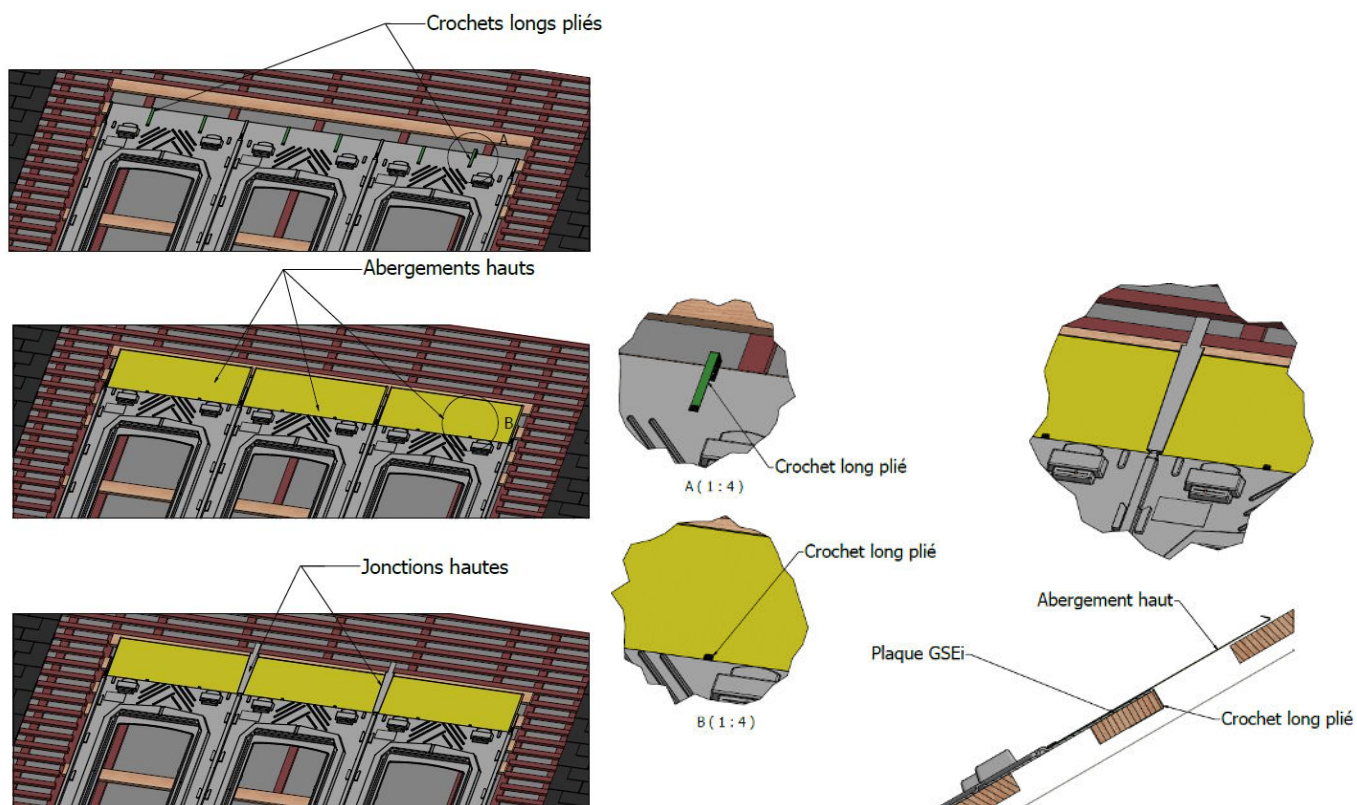
Figure 31 – Pose des abergements supérieurs (kit A-2)
