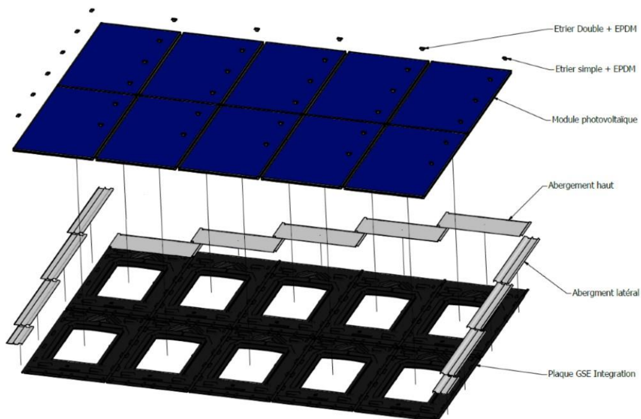
Figure 1 – Schéma éclaté du procédé
