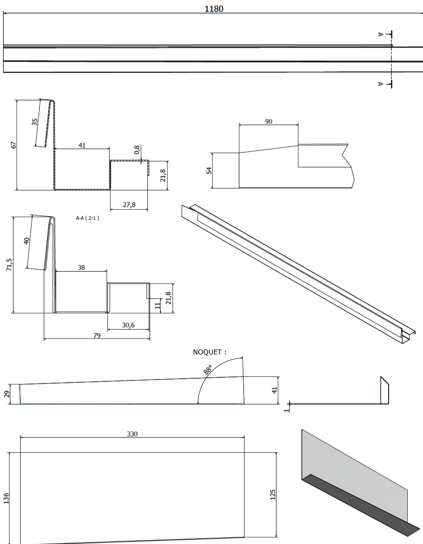
Figure 8 – Abergements pour kit A-2
