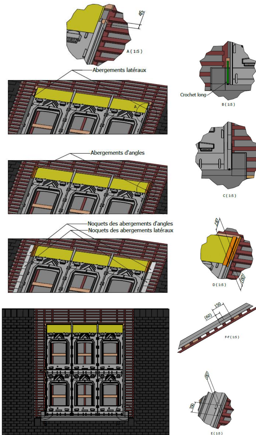
Figure 32 – Pose des abergements latéraux et d'angles supérieurs (kit A-2)
