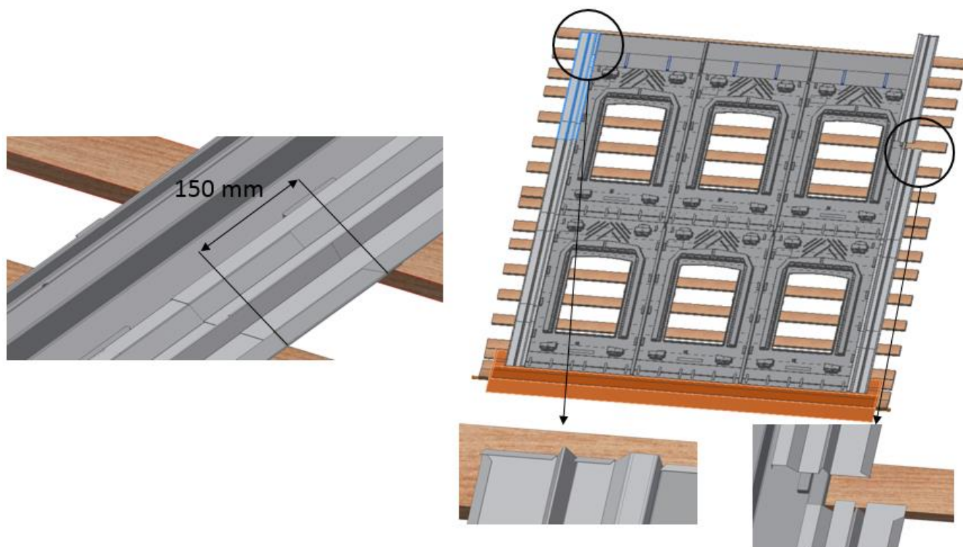
Figure 25 – Pose des abergements latéraux (kit TS-2)
