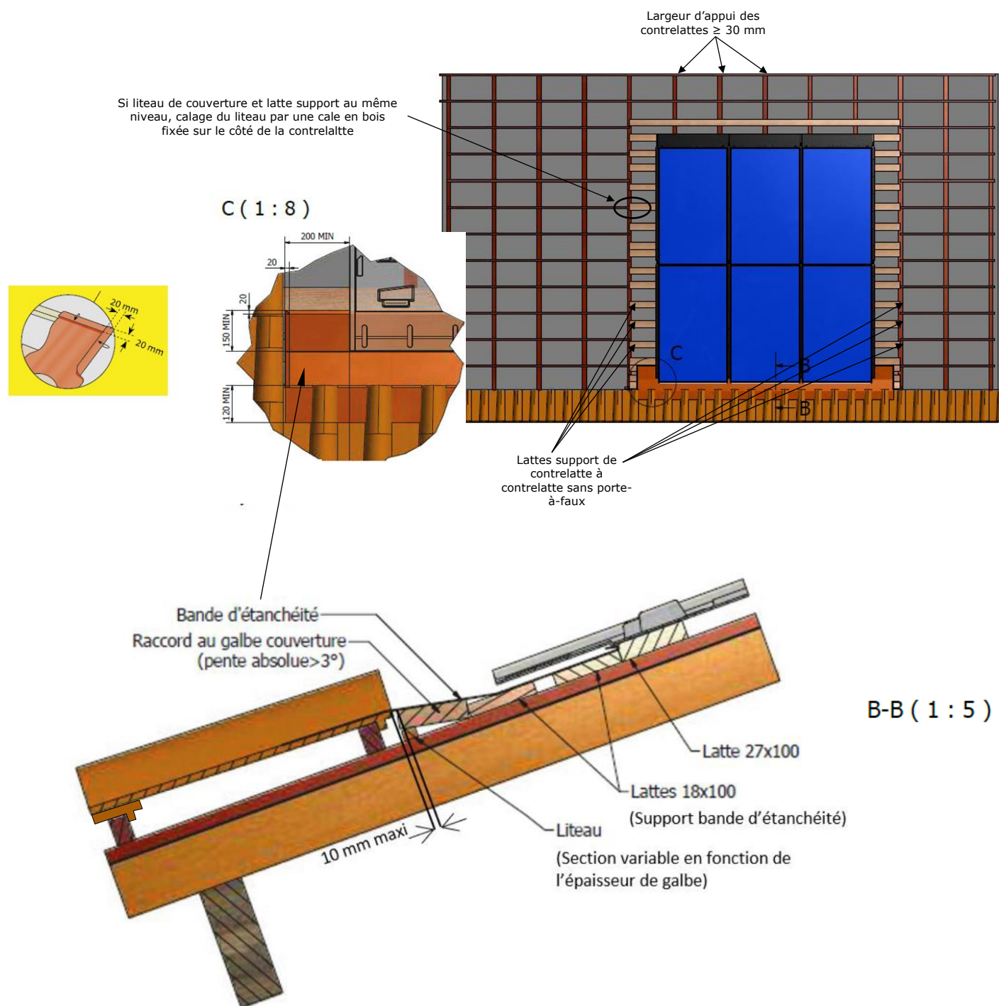
Figure 23 – Mise en œuvre du bas de champ (kit TS-2)
