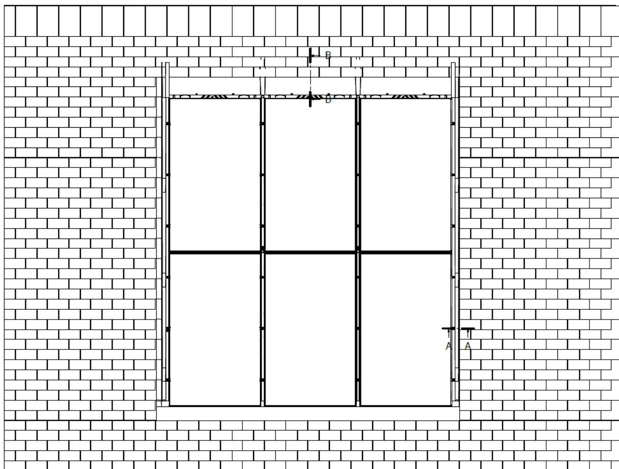
Figure 33 – Mise en place des éléments de couverture (kit A-2)
