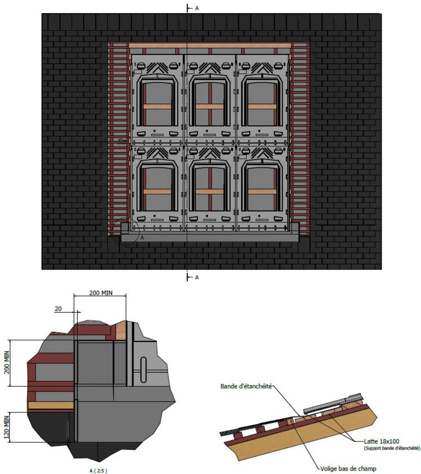
Figure 30 – Mise en œuvre du bas de champ (kit A-2)
