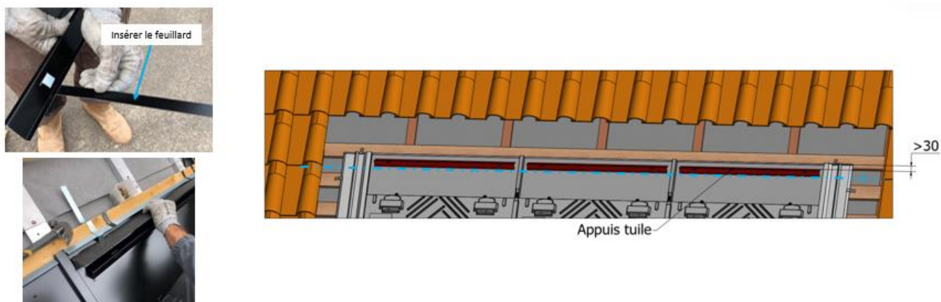
Figure 26 – Pose des appuis de tuiles (kit TS-2)
