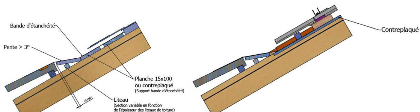
Pose de la bande en milieu de champ
