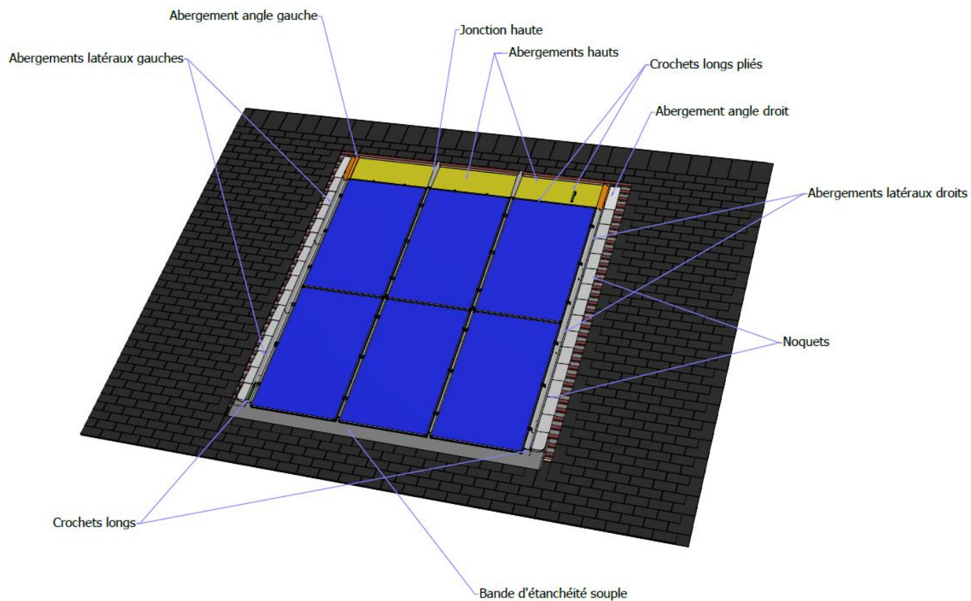
Figure 34 – Éléments du kit A-2 mis en œuvre
