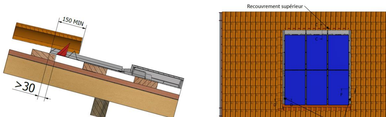
Figure 28 – Mise en place des éléments de couverture (kit TS-2)
