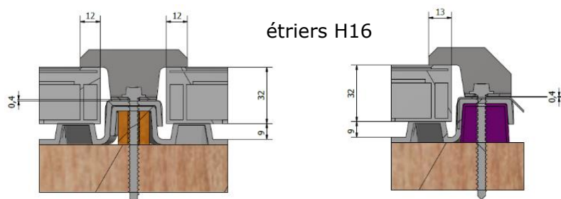
Figure 21 bis – Exemples de chaînes de cotes de l'écrasement du joint EPDM sous les étriers (suite) (il n'est pas possible de représenter tous les cas de figure)
