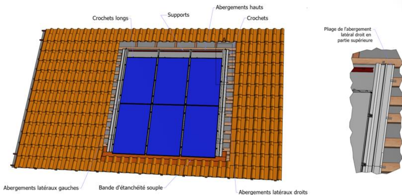
Figure 29 – Éléments du kit TS-2 mis en œuvre
