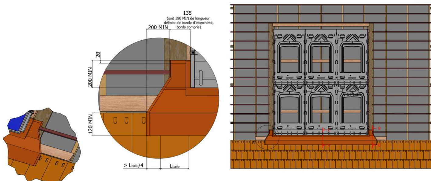
Pose de la bande en milieu de champ
