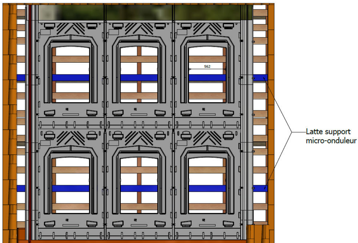
Figure 14 – Cas d'une mise en œuvre de micro-onduleurs
