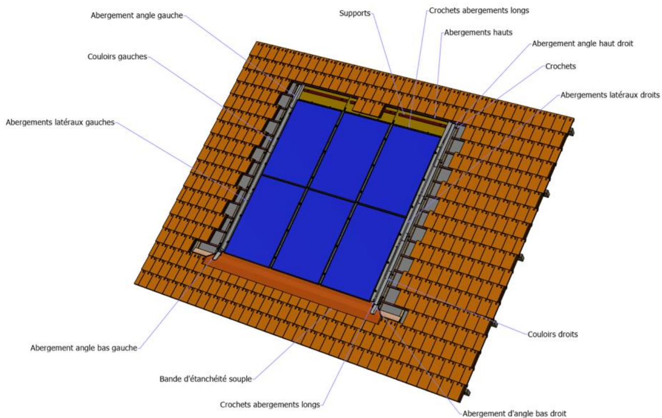
Figure 40 – Éléments du kit TN-1 mis en œuvre
