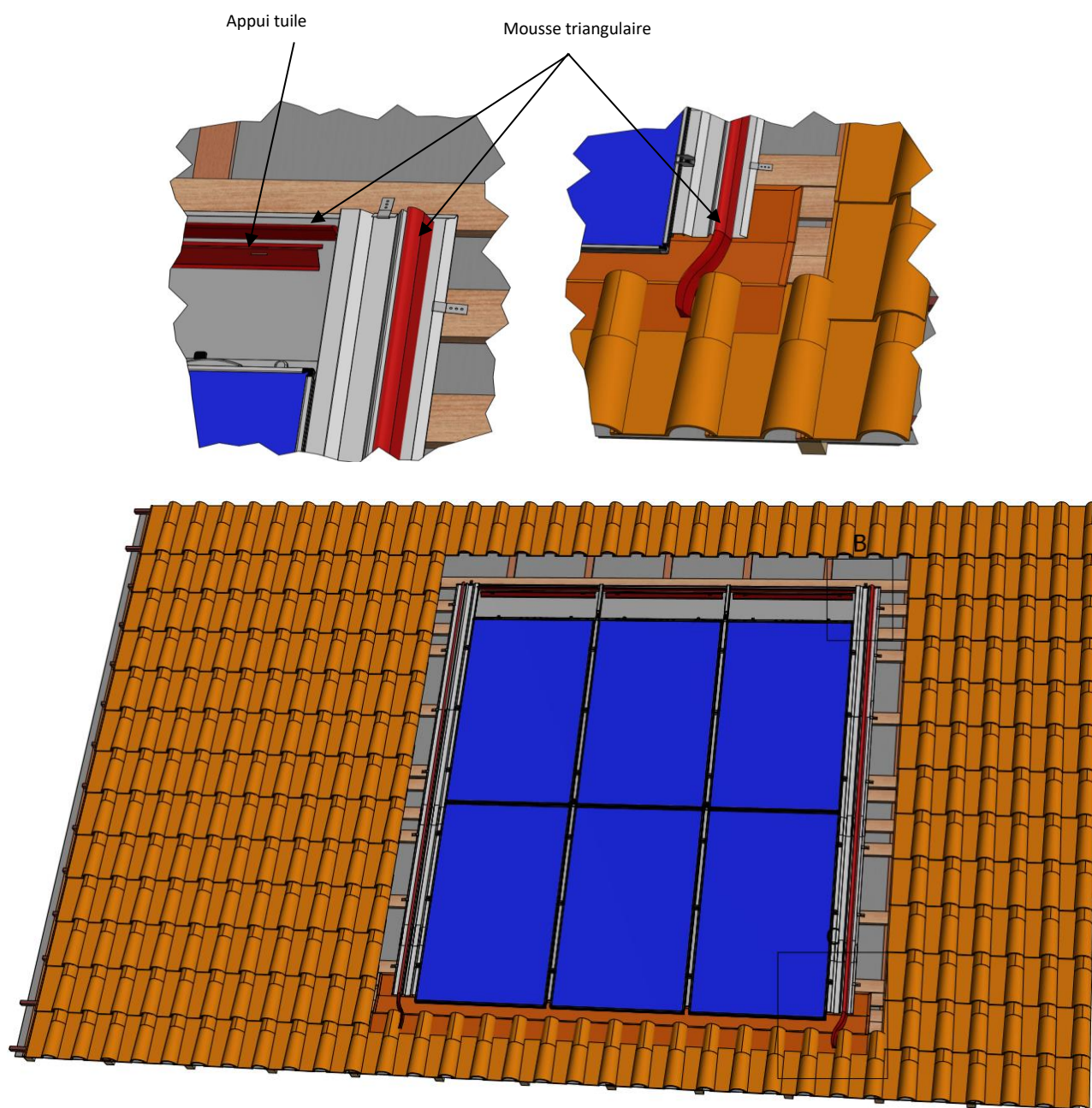
Figure 27 – Pose de la mousse triangulaire (kit TS-2)
