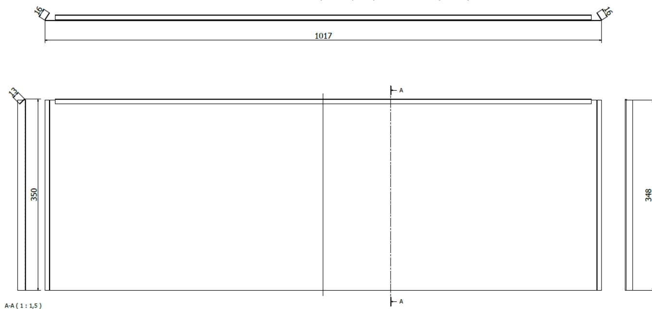
Figure 9 – Abergements supérieurs kit A-2
