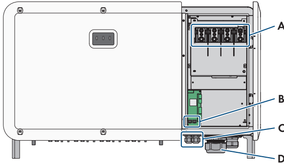
Figure 8 : Zones de raccordement situées à l'intérieur de l'onduleur
