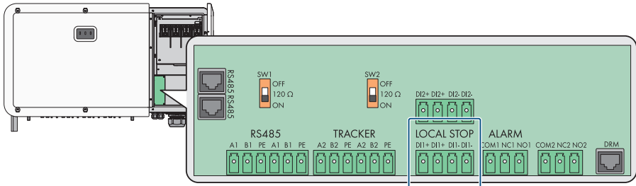
Figure 10 : Entrées numériques pour la fonction d'arrêt rapide sur l'ensemble COM
