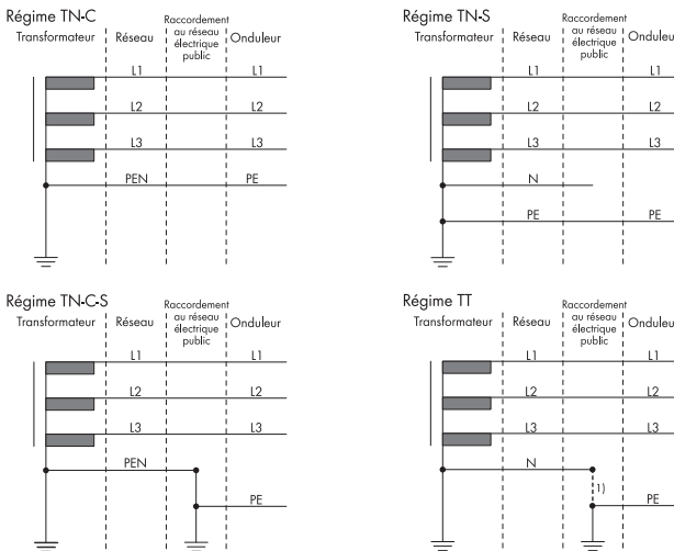
Figure 6 : Aperçu des schémas de liaison à la terre autorisés
