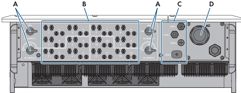
Figure 7 : Ouvertures du boîtier situées sur le dessous de l'onduleur
