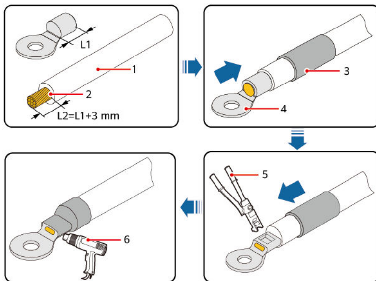
Figure 5-2 Sertissage d'une cosse OT
