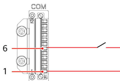
Figure E-1 Connexion des câbles à un commutateur d'arrêt rapide
